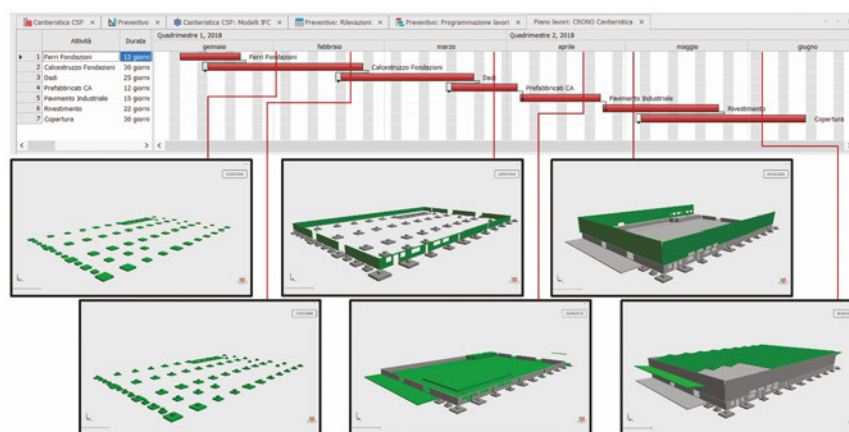
Simulazione 4D delle sequenze costruttive
